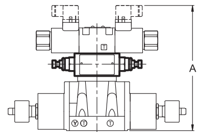
尺寸 mm
